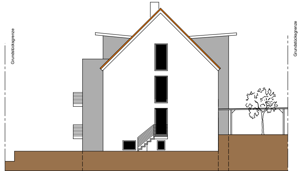
ANSICHT OST
