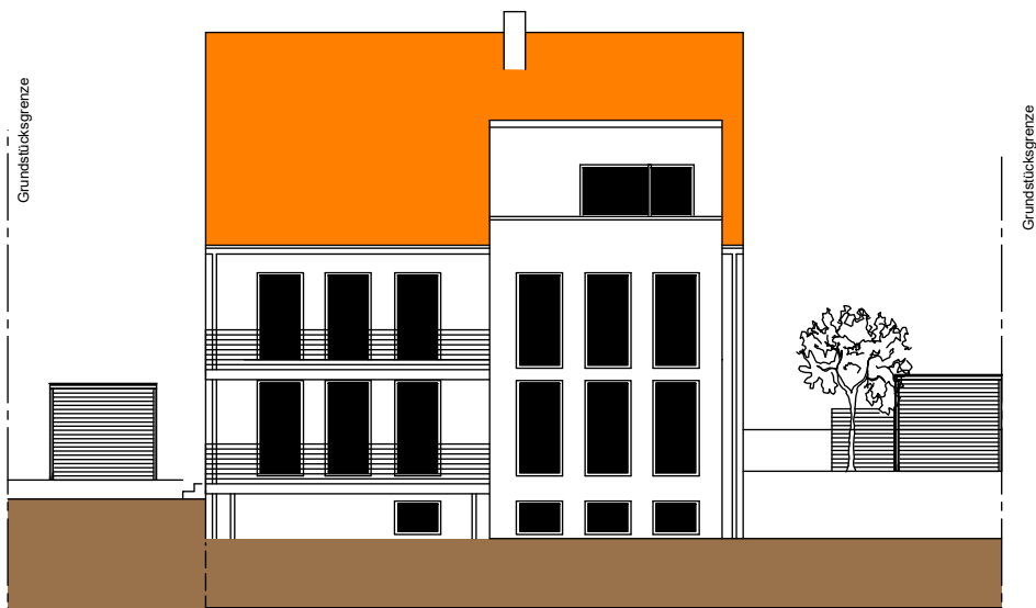
ANSICHT SÜD
